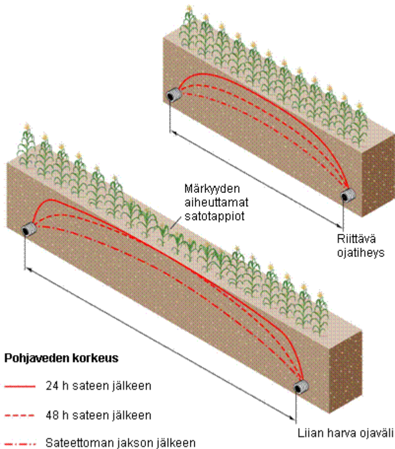
Kuva 17. Esimerkki salaoituksen ojavälin vaikutuksista kasvustoon. University of Illinois/ Salaojakeskus 2006.
