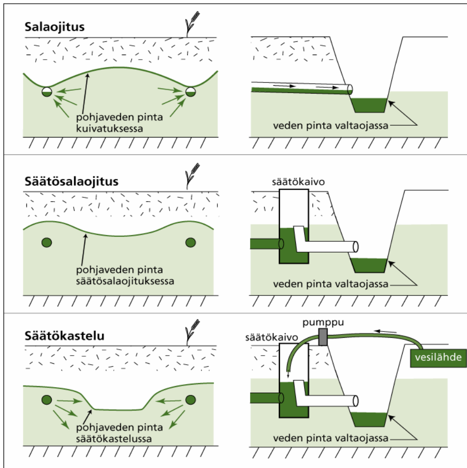
Kuva 12. Salaojituksen, säätösalaojituksen ja säätökastelun toimintaperiaatteet. Salaoja- keskus 2006.
