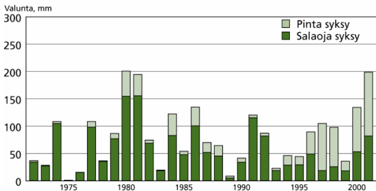
Kuva 8. Pinta- ja salaojavalunnat vaihtelevat merkittävästi eri vuosina. SYKE/Salaojakeskus 2006.
